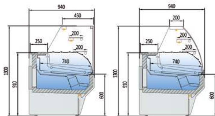
EVAPORADOR VENTILADO - VENTILATED EVAPORATOR
