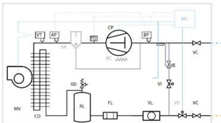
Esquema frigorífico DH - Centrífuga
