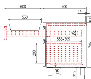
sin peto opcional optional, no splash-back
