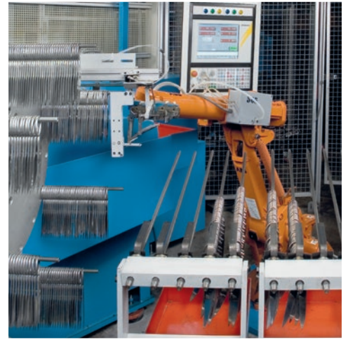
Amolado Grinding Meuleuse
